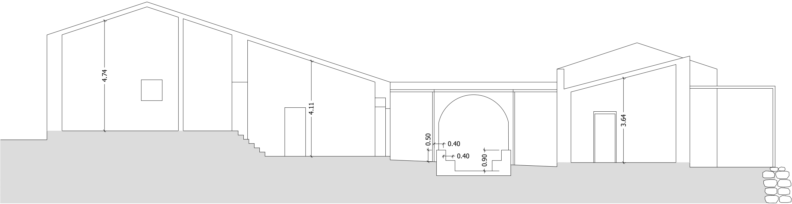
Sezione A_A
