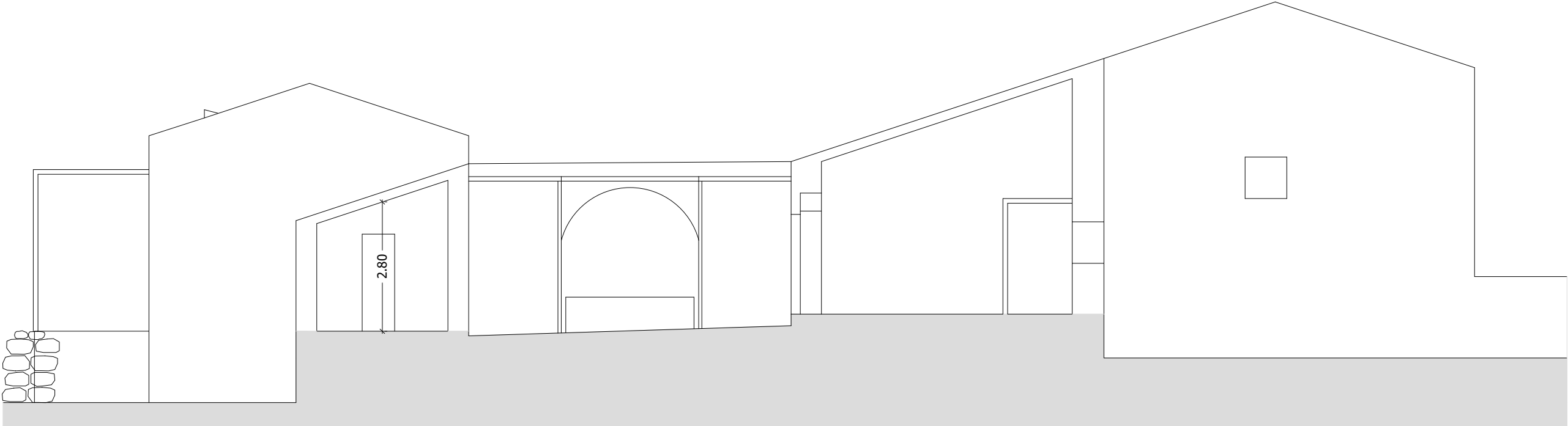
Sezione B_B
